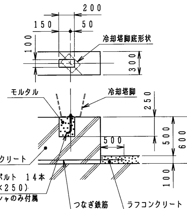
基礎参考図
