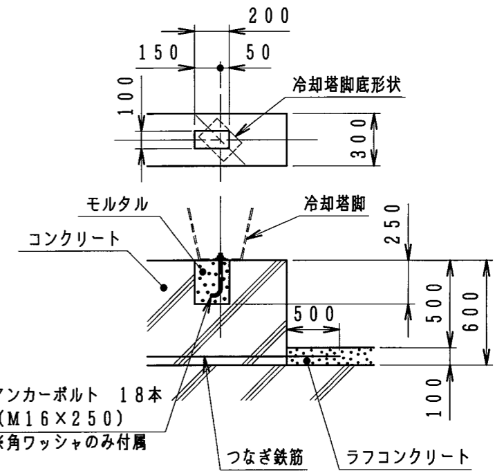
基礎参考図
