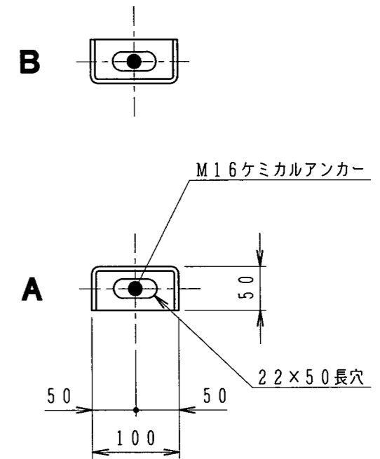
冷却塔脚部形状
