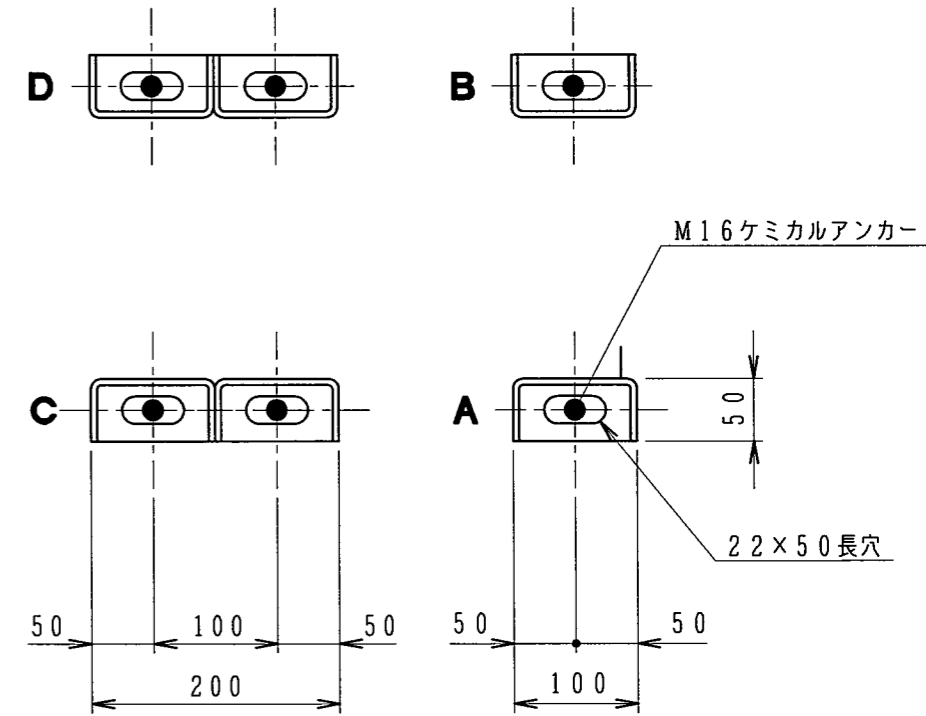
冷却塔脚部形状
