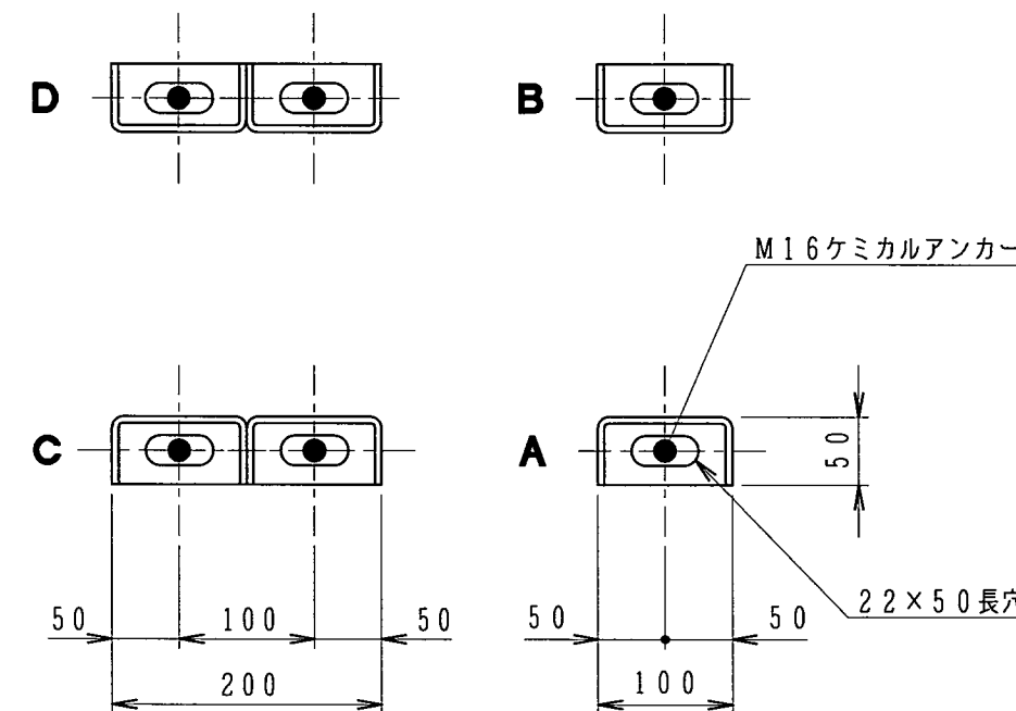
冷却塔脚部形状
