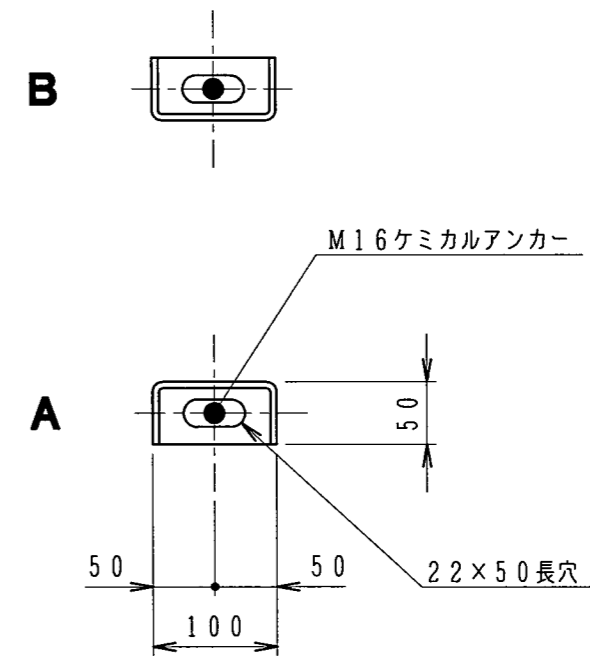
冷却塔脚部形状
