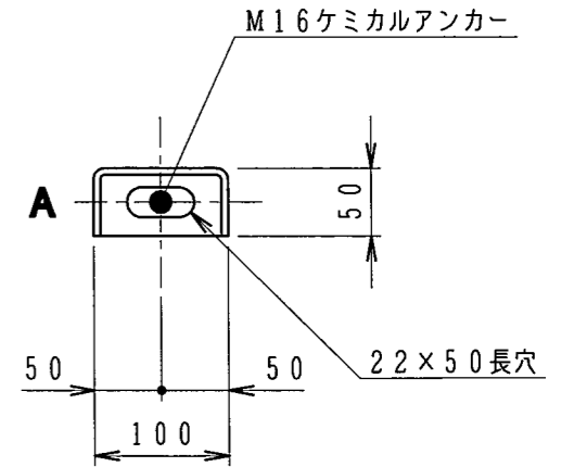
冷却塔脚部形状
