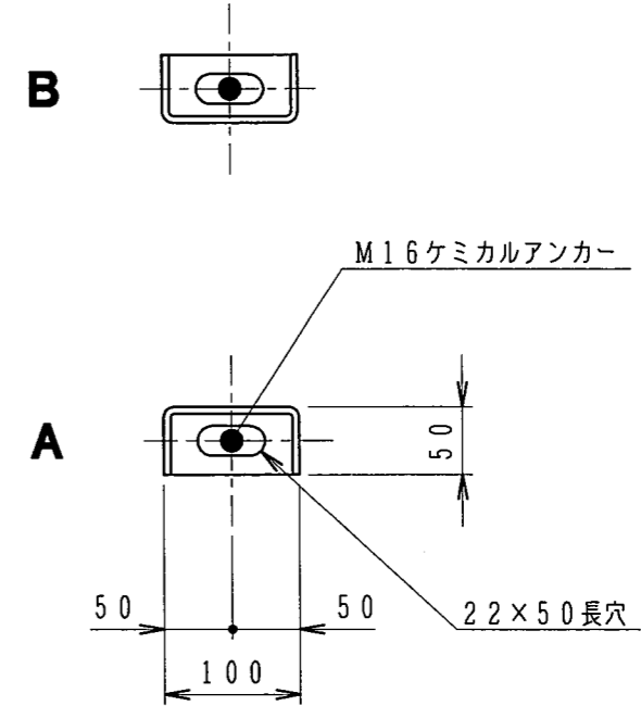
冷却塔脚部形状
